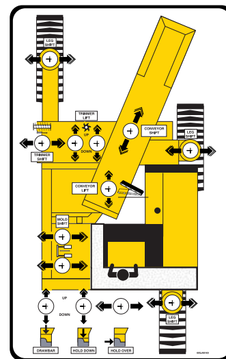
Панель управления трехгусеничной машины
